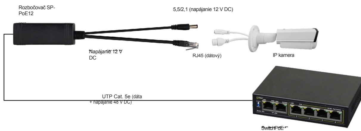
Obr. 2. Príklad pripojenia k PoE prepínaču.
