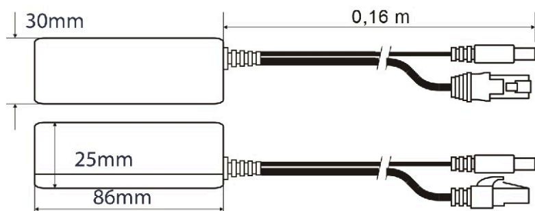
Obr. 1. Mechanický pohľad.
